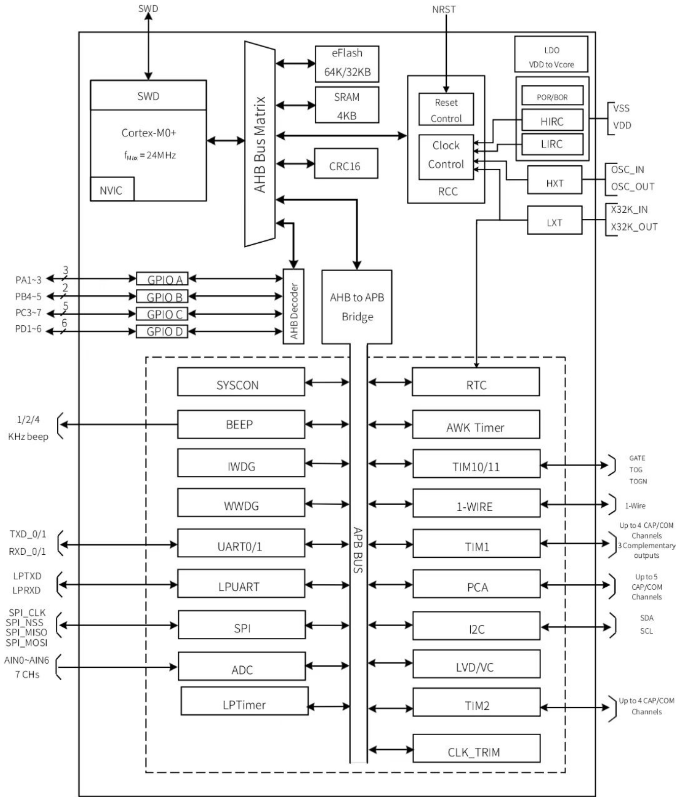
图 1 系统框图
