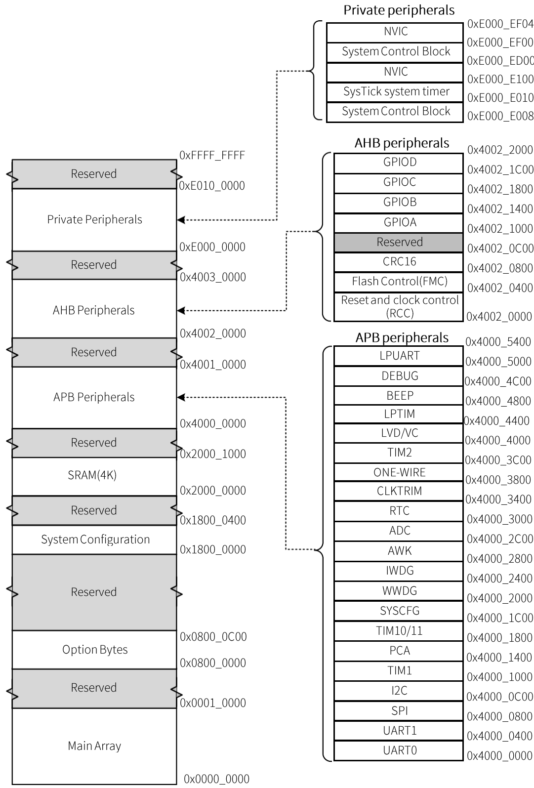
图 2 内存映像
